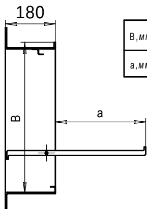
Рис. 2. Вылет заслонки за пределы корпуса клапана
